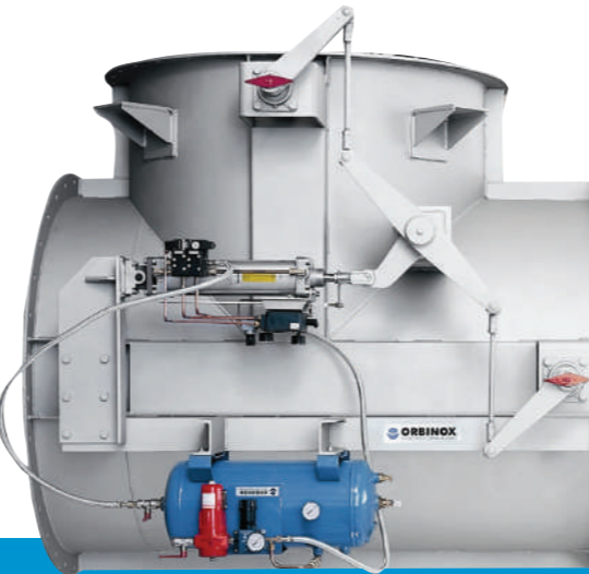
DI Distribuidor de gases Multiple diverter damper 3-Wege Klappe
